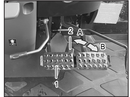
(1) 브레이크 페달 (2) 연결판 (A) 해제 (B) 연결
